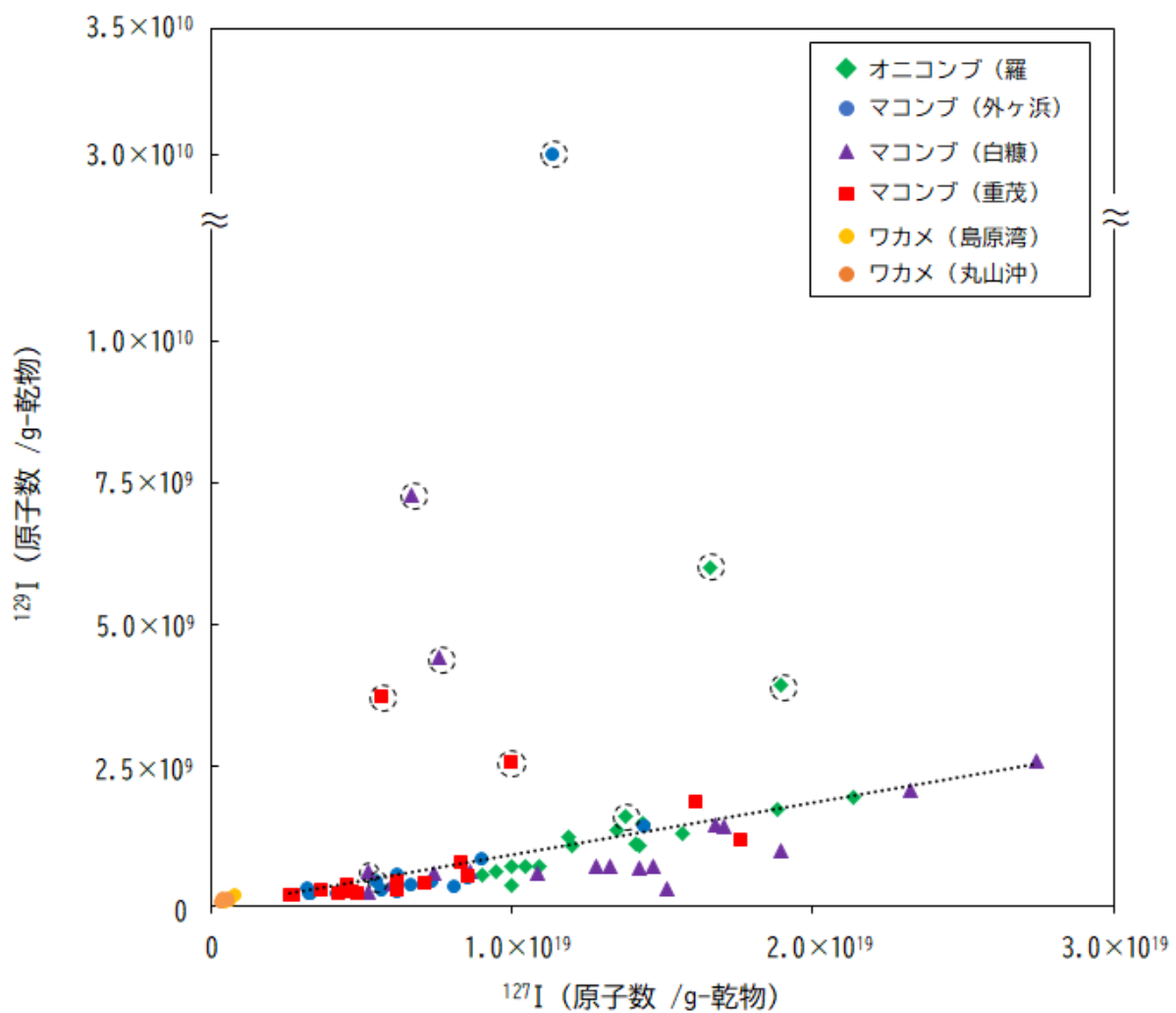
図 I-2-3-2-7 平成 19 年～令和 6 年までに得られた海藻試料に含まれる ^{127}\text{I} と ^{129}\text{I} の関係 (図中の回帰直線は、点線で囲まれたアクティブ試験 (平成 19～20 年) 及び東電福島第一原発事故 (平成 23 年) の影響がある 10 試料を除いたコンブ類試料のみで計算した。)
