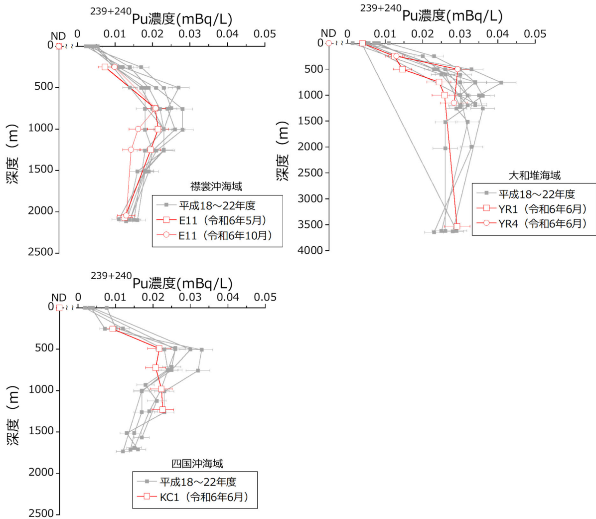
図 I -2-2-1-4 対照海域で採取した海水試料に含まれる ^{239+240}\text{Pu} 濃度の鉛直分布（誤差棒は計数誤差を示す。また、NDは検出下限値未満を示す。）
