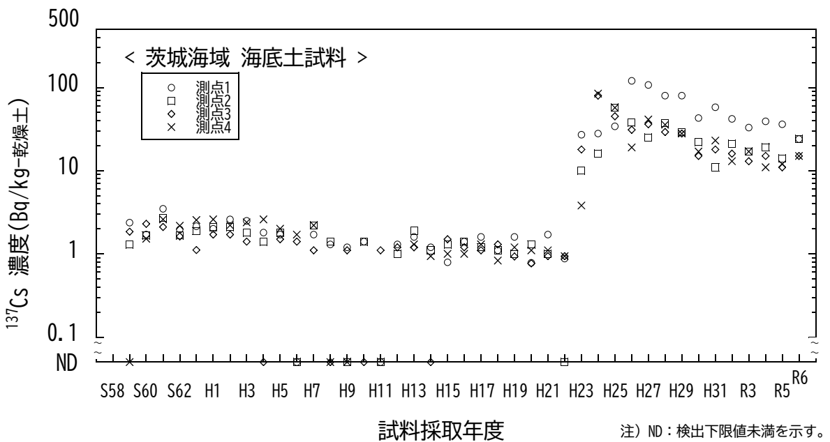
図 I-1-6-19 海底土試料の ^{137}\text{Cs} 濃度の経年変化 (茨城海域)
