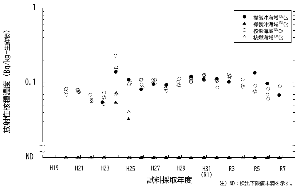
図 I -2-2-2-6 対照海域（襟裳沖海域）及び核燃海域で収集したシロザケに含まれる ^{134}\text{Cs} 及び ^{137}\text{Cs} 濃度の経年変化
