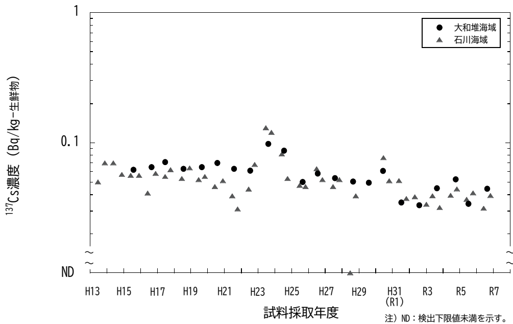
図 I-2-2-2-3 対照海域(大和堆海域)及び石川海域で収集したホッコクアカエビに含まれる ^{137}\text{Cs} 濃度の経年変化
