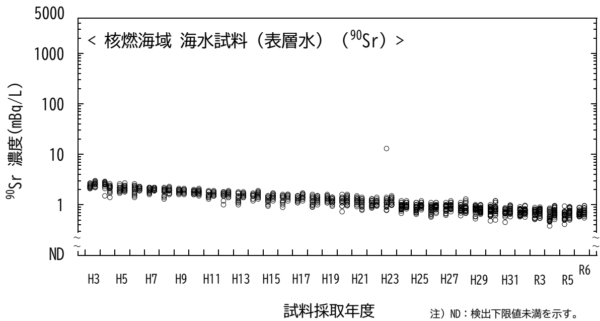
図 I-1-6-66 海水試料の ^{90}\text{Sr} 濃度の経年変化（核燃海域・表層水）
