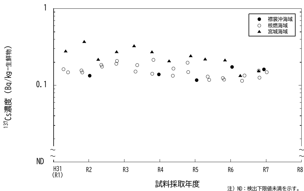
図 I-2-2-2-5 対照海域（襟裳沖海域）、宮城海域及び核燃海域で収集したマダラに含まれる ^{137}\text{Cs} 濃度の経年変化
