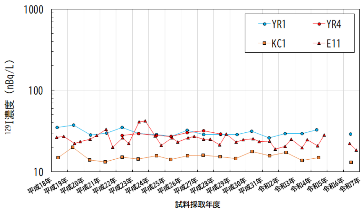
図 I-2-3-2-3 対照海域の表層水に含まれる ^{129}\text{I} 濃度の時系列変化
