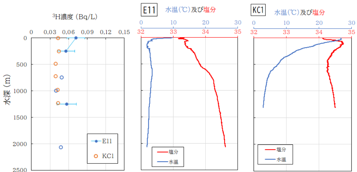
図 I-2-3-3-2 対照海域で採取した海水試料に含まれるトリチウム濃度、採水容器に取り付けた機器により連続観測を行った塩分及び水温の鉛直分布 (トリチウムが検出されなかった試料は白抜きとし、検出下限値を代入した。)
