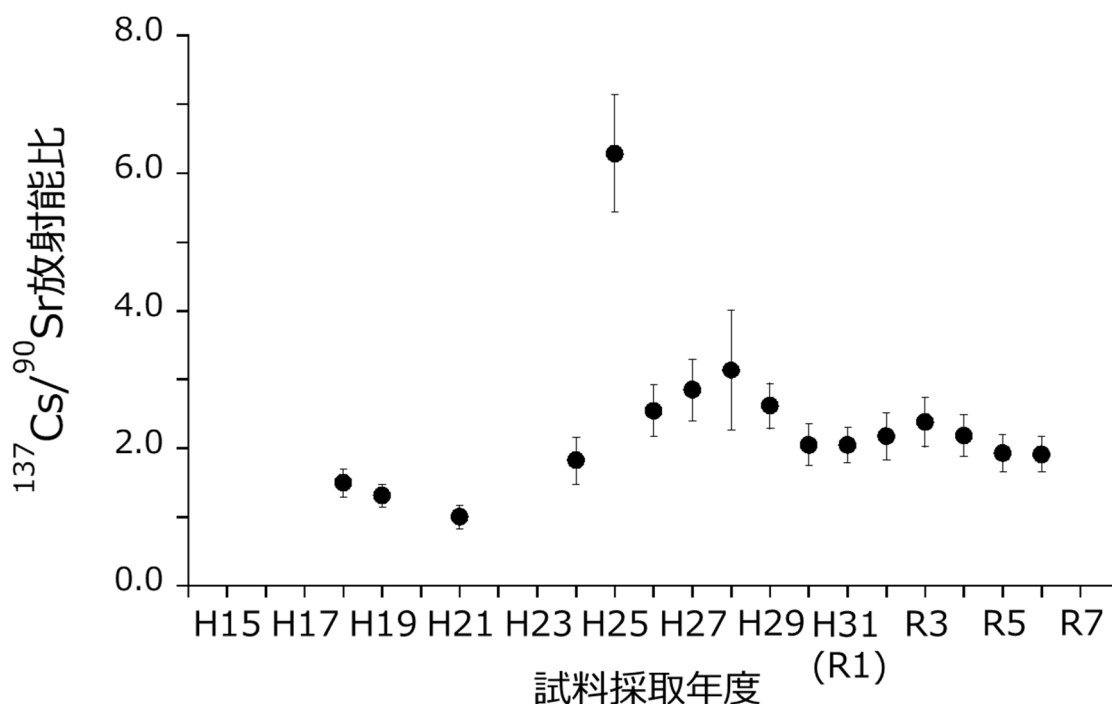
図 I -2-2-1-6 対照海域（四国沖海域）の深度 250 m 付近で採取した海水試料の ^{137}\text{Cs}/^{90}\text{Sr} 放射能比の推移（誤差棒はそれぞれの計数誤差を伝播して得られた数値を示す。なお、平成 24～25 年度の ^{137}\text{Cs}/^{90}\text{Sr} 放射能比は極低バックグラウンドガンマ線スペクトロメトリーにより定量した ^{137}\text{Cs} 濃度を用いて算出した。）
