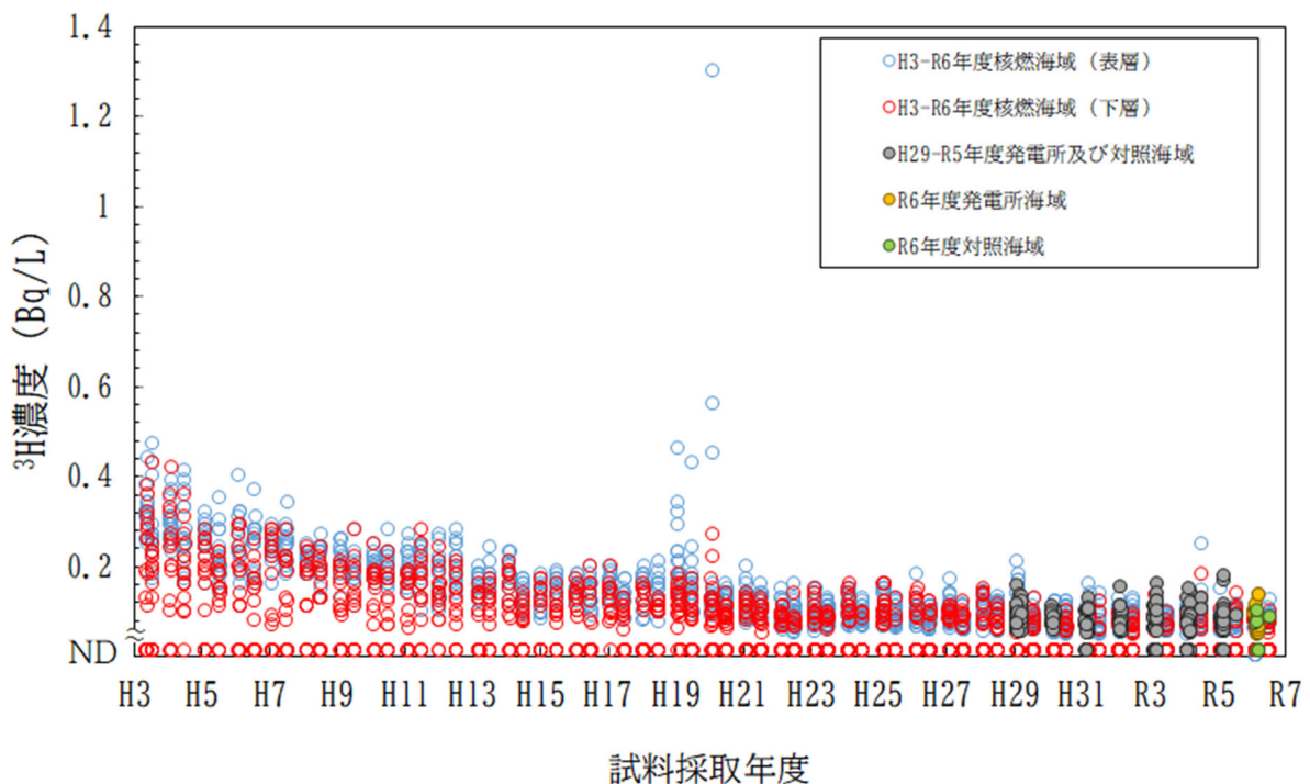
図 I-2-3-3-3 海水試料に含まれるトリチウム濃度の経年変化（ND は検出下限値未満を示す。）
