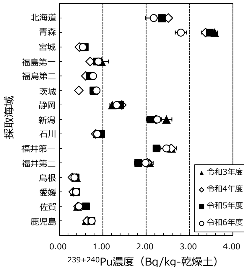
図 I -2-3-1-1 発電所海域で採取した海底土試料に含まれる ^{239+240}\text{Pu} 濃度
